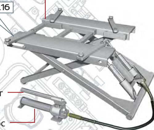
Подъемник гидравлический
